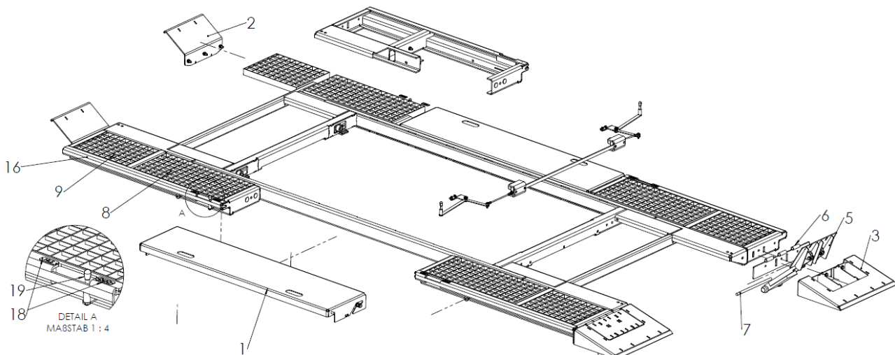
Explosionsansicht - Ausleger HLS3513-DUO-11
