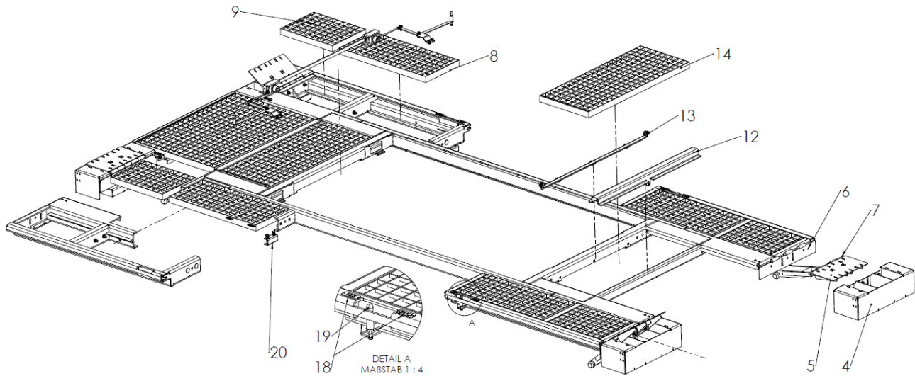
Explosionsansicht - Ausleger HLS3513-DUO-14
