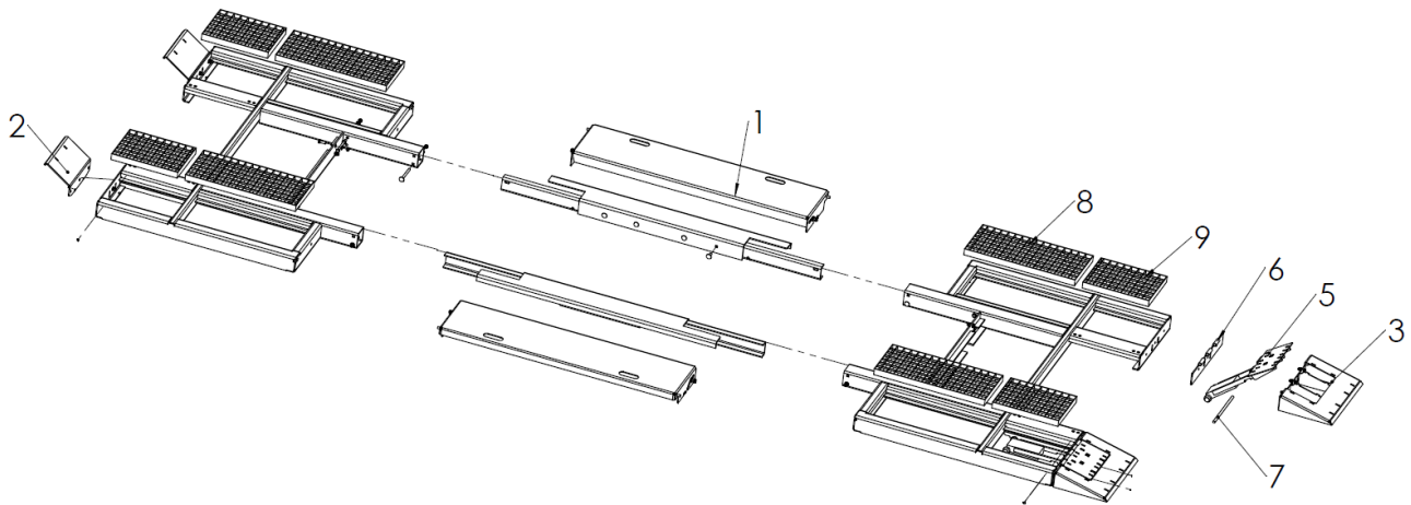
Explosionsansicht - Ausleger HLS3513-11
