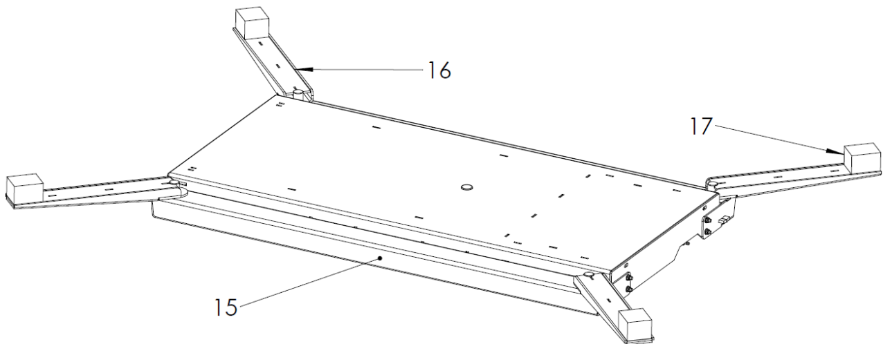
DUO-Anbauteile für Grundkörper HLS3513-DUO-11 & HLS3513-DUO-14 HM-Anbauteile für Grundkörper HM3513-01 & HM3513-04
