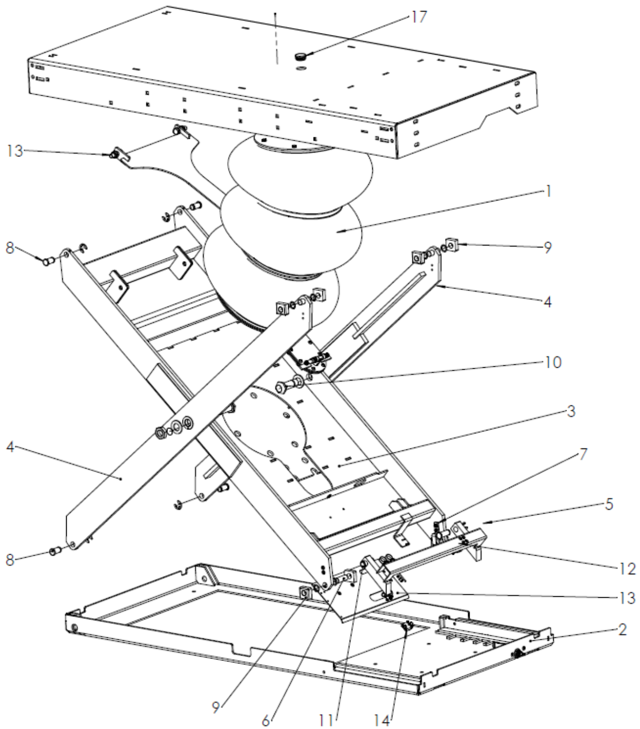
Explosionsansicht - Grundkörper K3513
