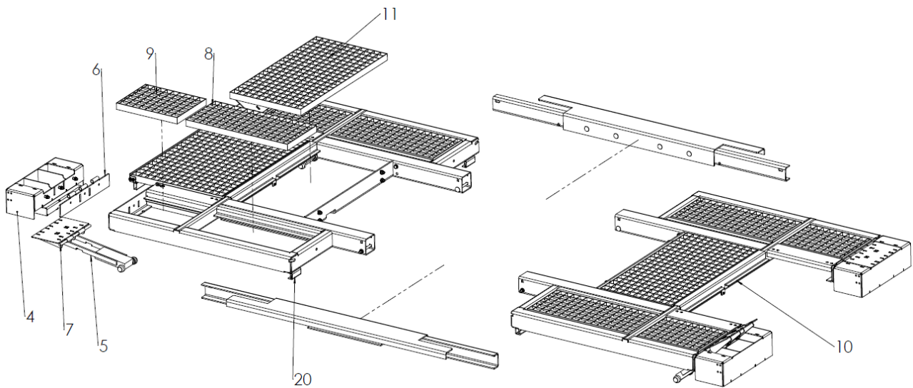
Explosionsansicht - Ausleger HLS3513-14
