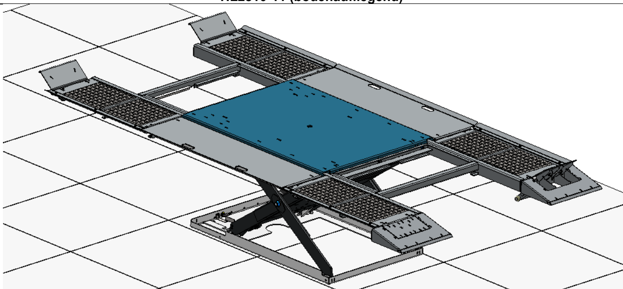
HL2810-11 (bodenauflegend)
