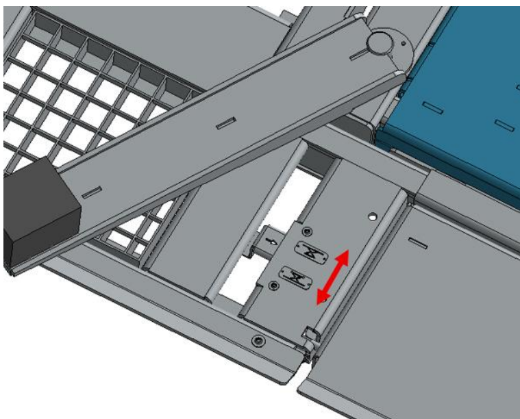
entkoppelt (radfreihebend)
