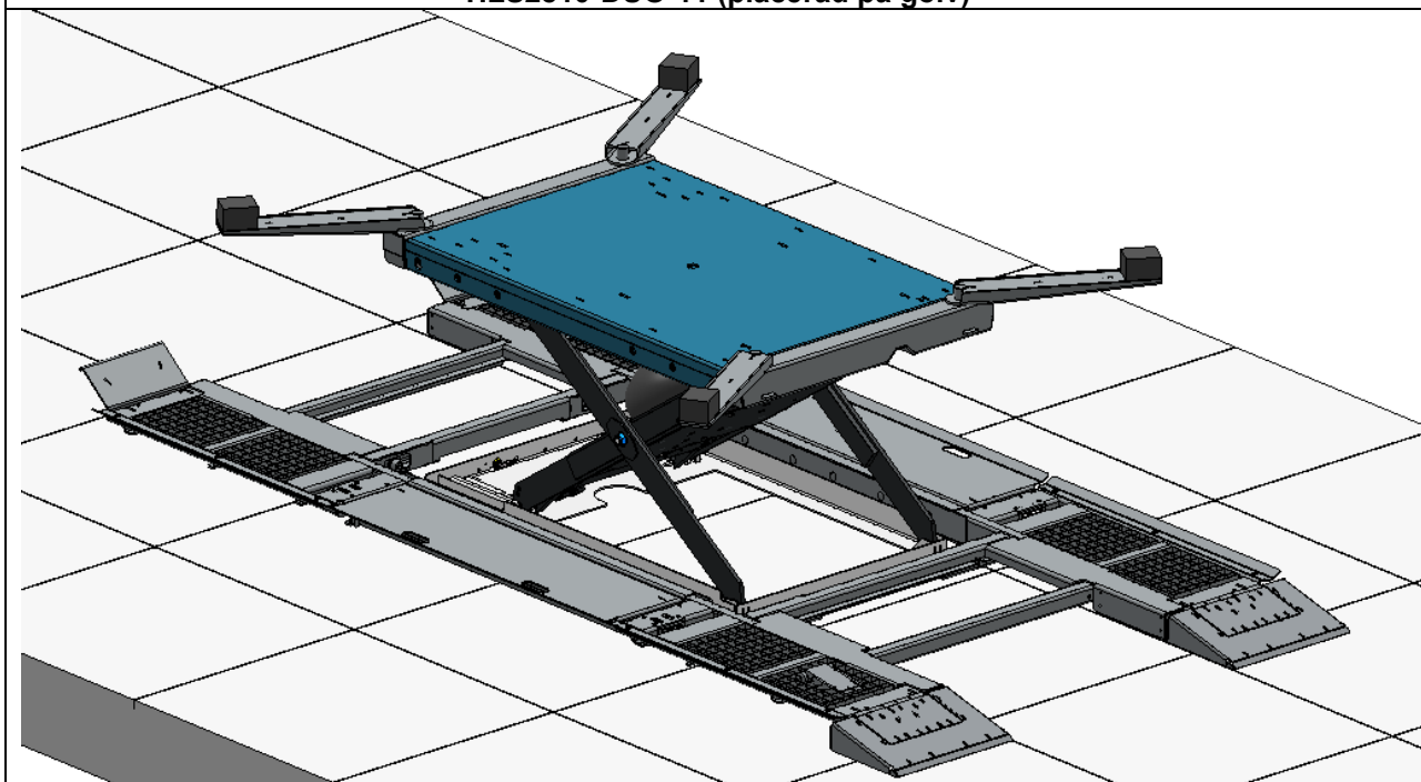
HLS2810-DUO-11 (placerad på golv)
