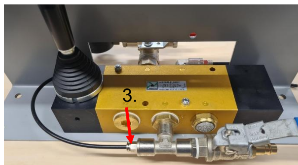
3. Ø4 PA-slang
