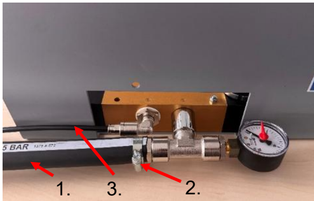
1. 15er Gummischlauch 2. Schlauchschelle
