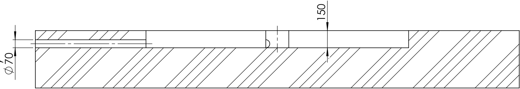
SCHNITT A-A
