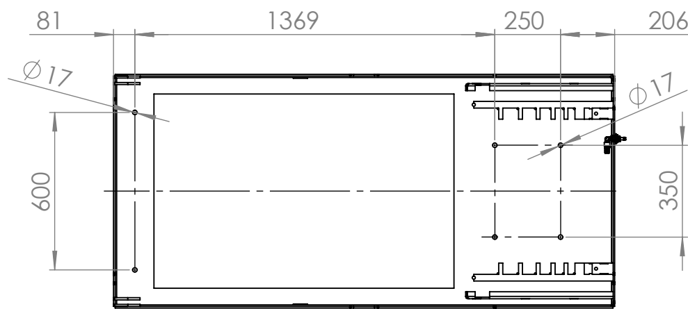
Bodenverschraubung/Bottom screwing
