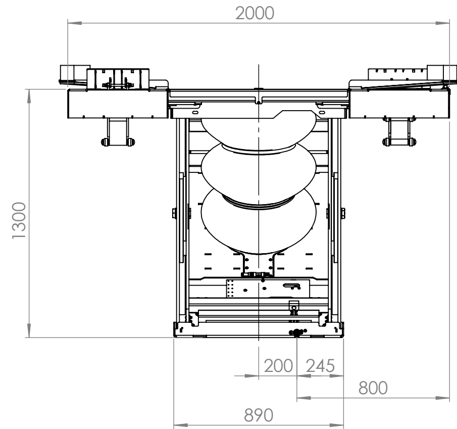
Bodenverschraubung/Bottom screwing
