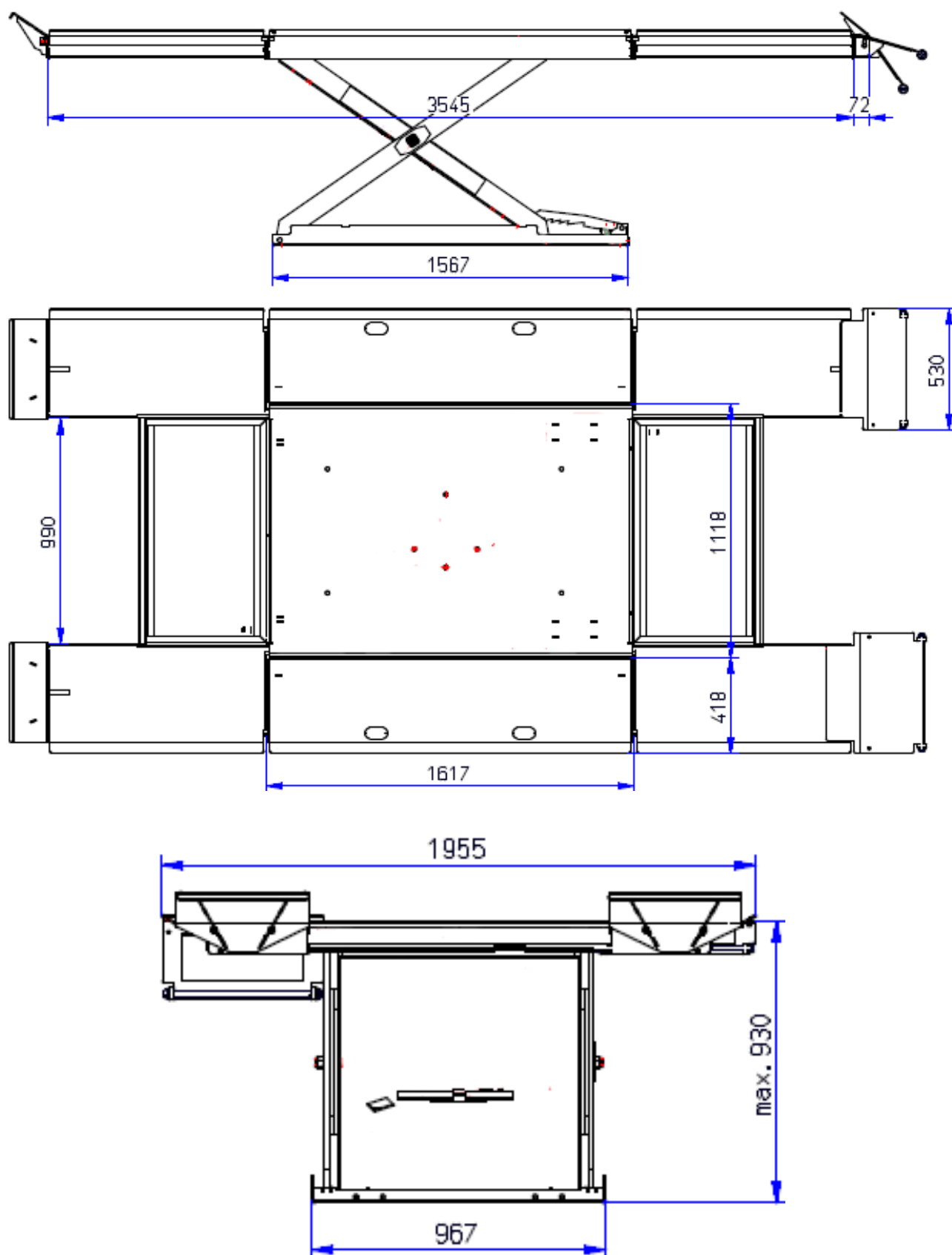
Maßblatt HLS1200-14 und HLS1200-16
