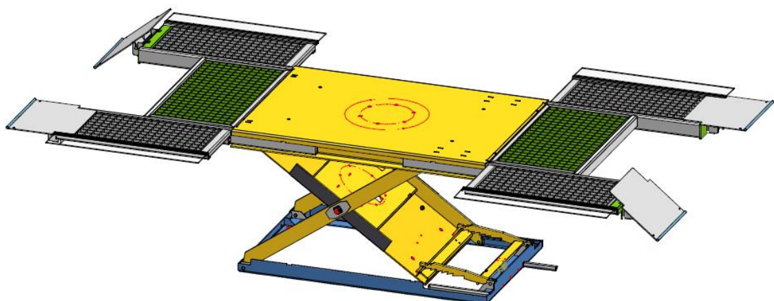
Bild 2: Produkt HLS1200-14 / -16
