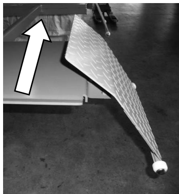
Image 6 : Table élévatrice en position haute avec rampe de montée installée
