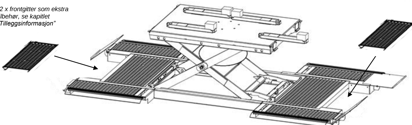
Fig. 2: Produktet HLS1200-DUO-14
