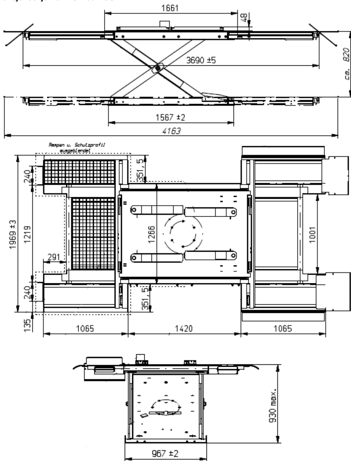
Dimensjonsskjema HLS1200-DUO-14
