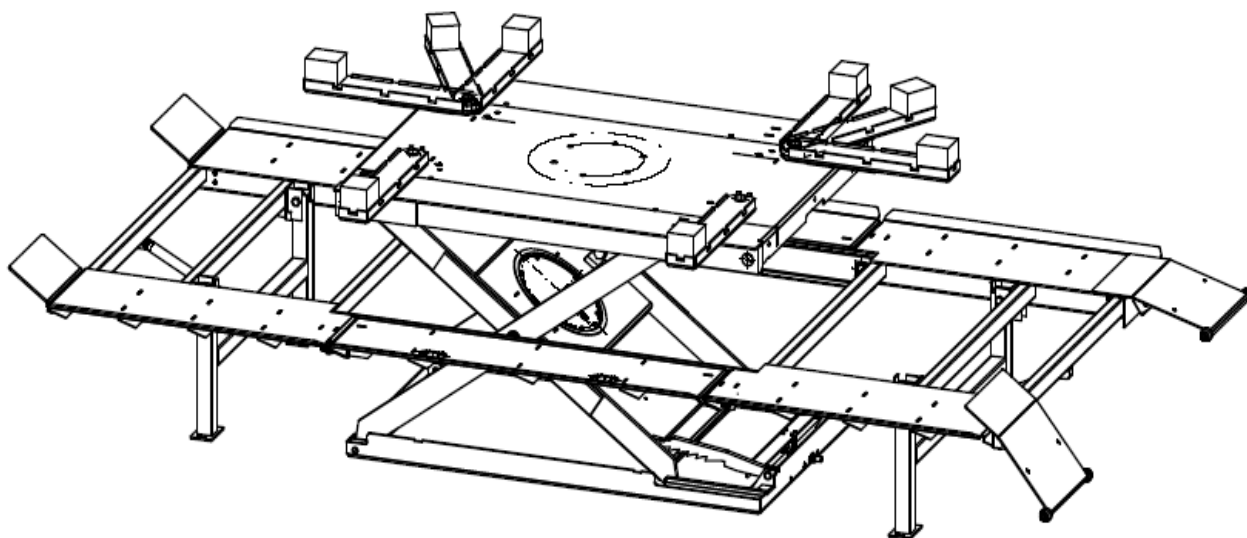
Fig. 1: Produktet HLS1200-DUO-11
