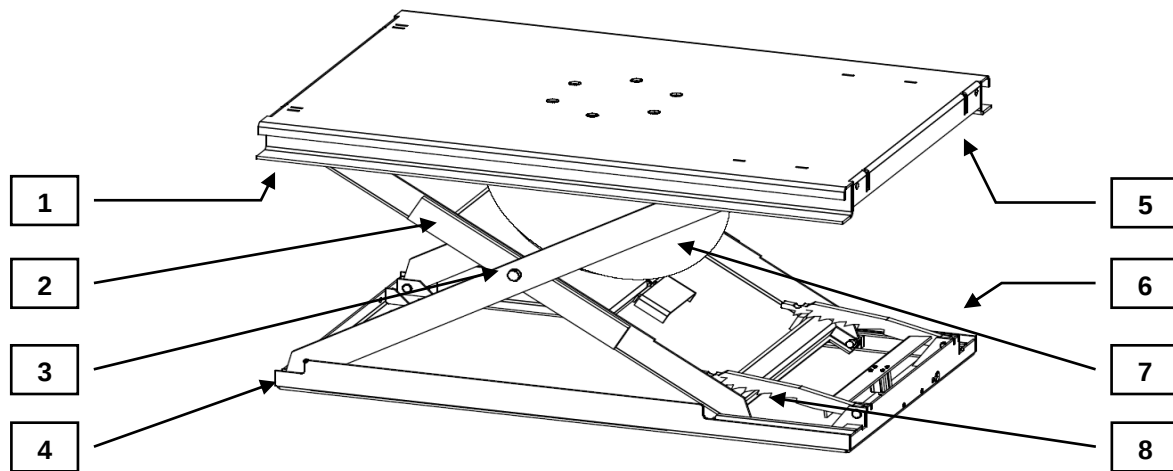
Bild 16: Prüf- und Schmierpunkte
