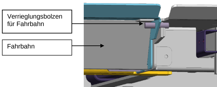
Bild 9: Fahrbahn aus-/eingeklappt und verriegelt
