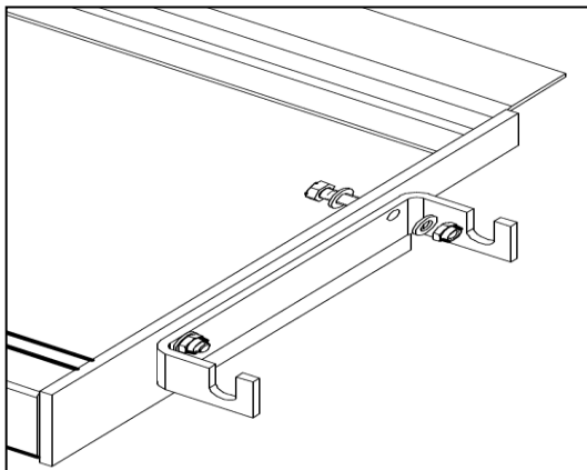
Bild 6: Rampenhalter und Auffahrrampe montieren
