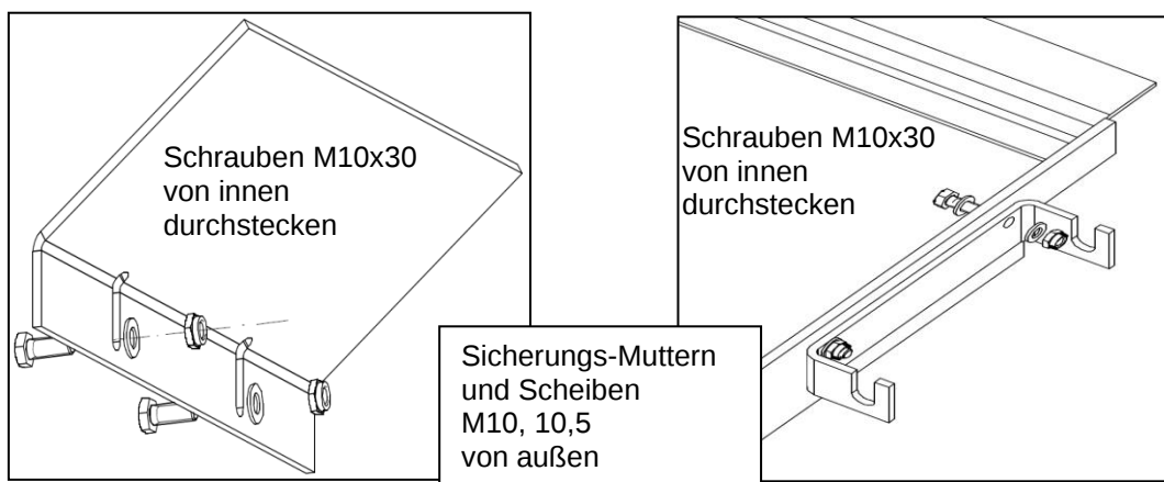
Bild 2: Überrollschutz montieren
